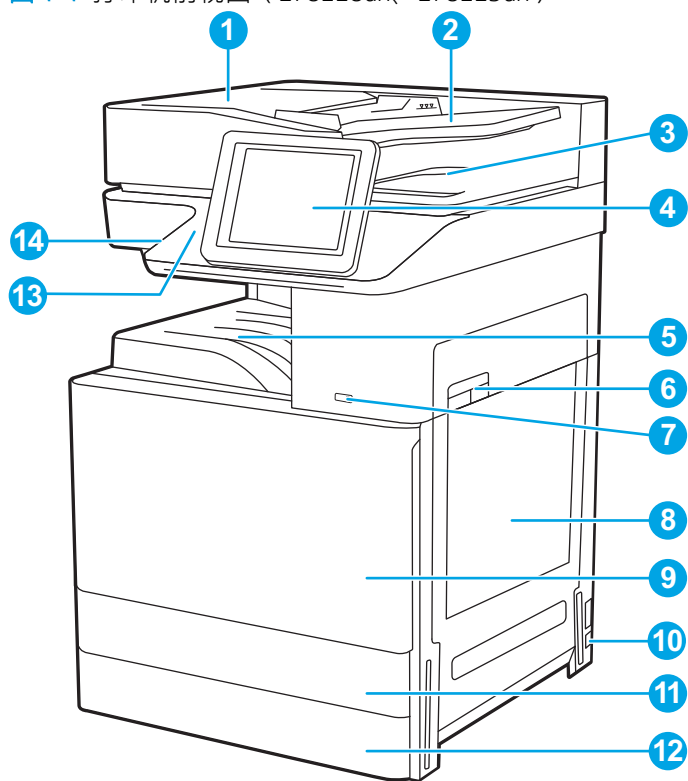
图 1-1 打印机前视图 (E78228dn、E78223dn)
