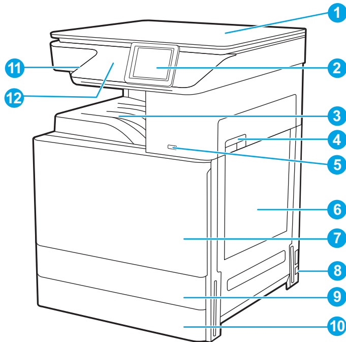
图 1-3 打印机前视图 (E78223a)
